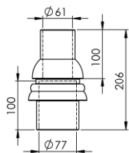
REDUSER Ø76 - Ø 60
