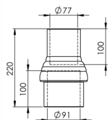
REDUSER Ø90 - Ø 76
